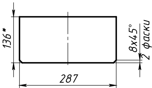
Поз.3 (Ребро среднее)
