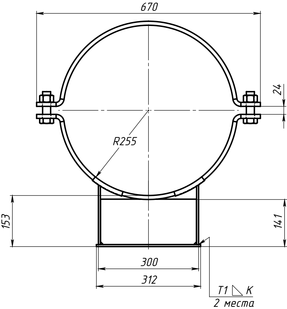
Поз.4 (Полухомут)
